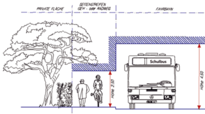
Freizuhaltenes Lichtraumprofil an öffentlichen Straßen, Wegen und Plätzen
